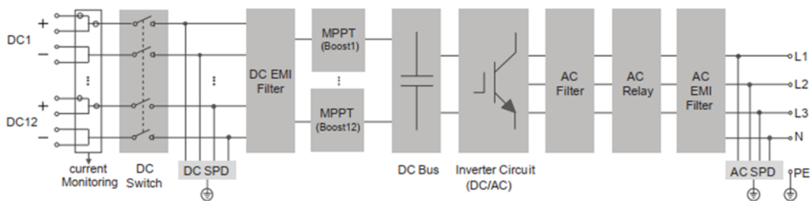
Εικόνα 3.2.1 Χαρακτηριστικά αντιστροφέα ενδεικτικού τύπου (125kW) (α)
