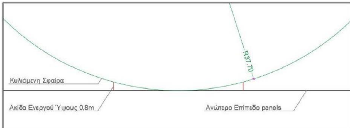
Εικόνα 7.3.1 Υπολογισμός ελάχιστης ακτίνας κυλιόμενης σφαίρας για απόσταση ακίδων 15μ.
